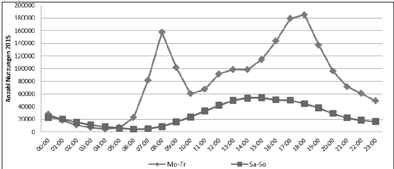
Tagesganglinie 2015
